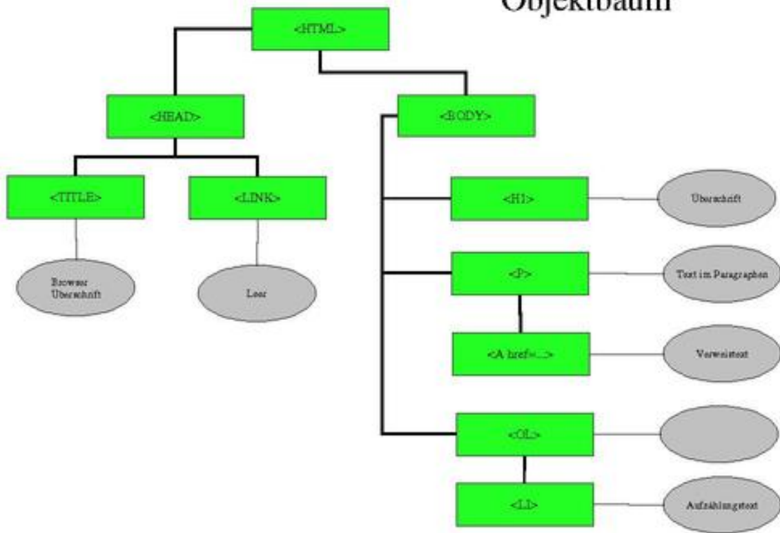
Objektbaum nach dem Parsen
